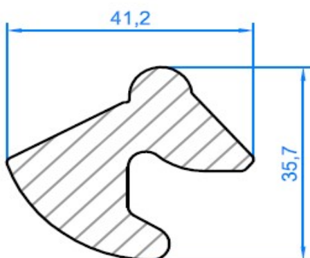
Profil pour barre antipanique Anti-panic bar profile Profil für Anti-Panikstange
