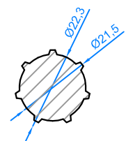
Spur section Arbre
