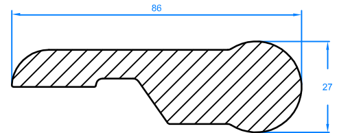
Hinge Profile Profil charnière pour compas
