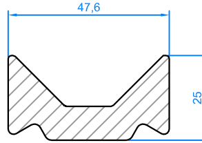
Profile for matrix Profil pour matrice
