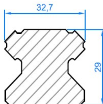
Profil de guidage Linear bearing Führungsschiene
