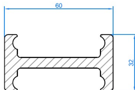
Rail de guidage Linear ball rail Führungsschiene
