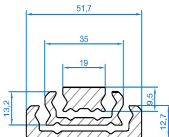
Glissières télescopiques Telescopic slides Teleskopschienen
