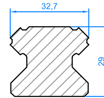
Linear bearing Profil de guidage
