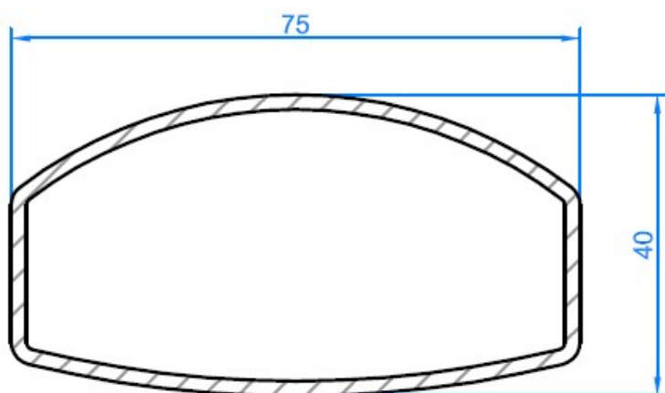
Barre de guidage Fork lift drawbar Deichsel eines Gabelstaplers
