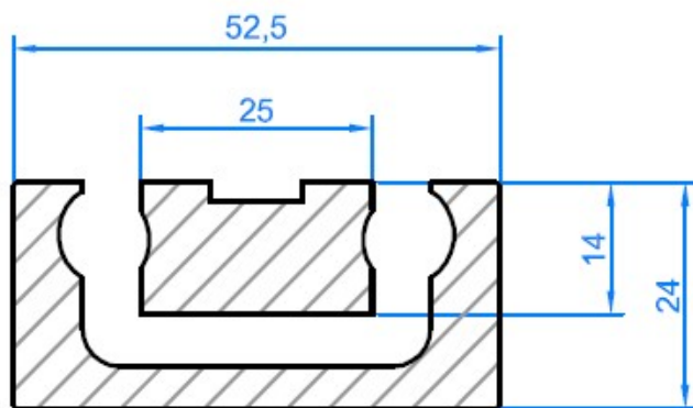
Guidage porte de train Train door track Zugtürführung
