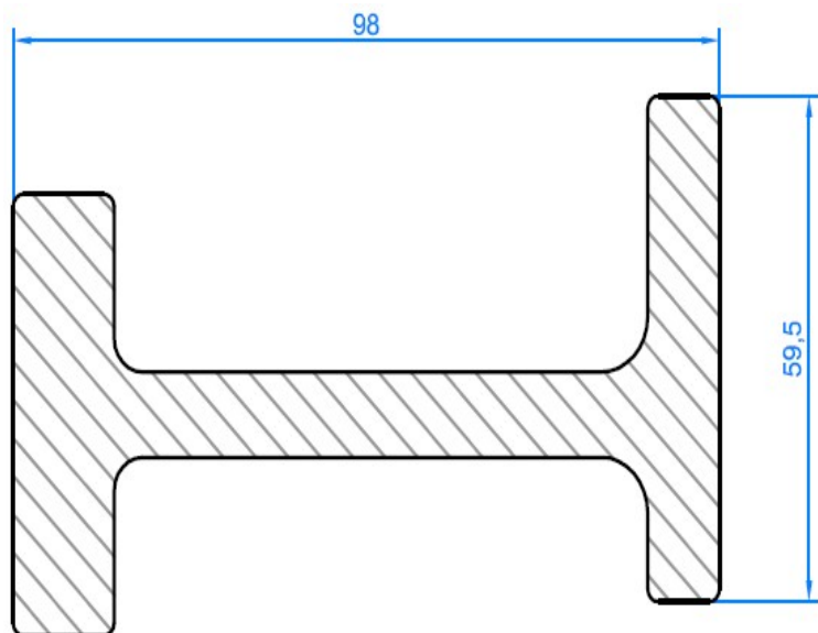
Profil pour chariot élévateur Fork lift section Profil für Gabel-Stapler
