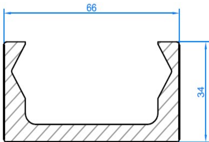
Rail de porte de train Train door track Schiene für Zugtüren
