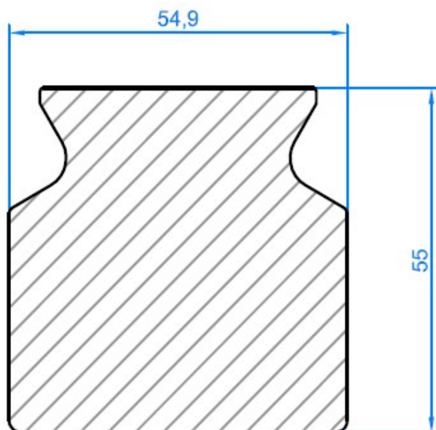
Profil pour générateur Generator stator profile Profil für Generator
