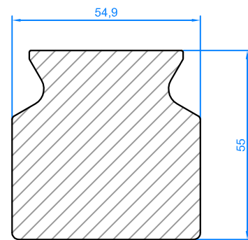
Profile for generator stator Profil pour générateur
