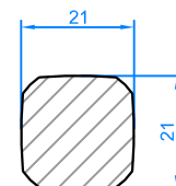
Polygon shaft Arbre polygon
