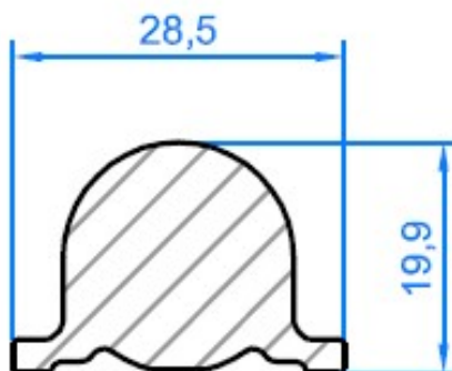
Gachette Trigger Auslöser
