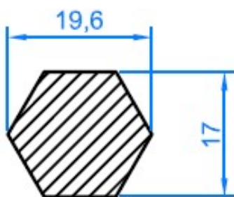
Barre de torsion portes pour char Leclerc Doors torsion bar for Leclerc tank Türen-Torsionsstange für Leclerc Panzer
