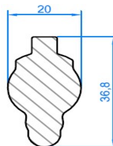
Corps de pistolet Pistol body Pistolenkörper
