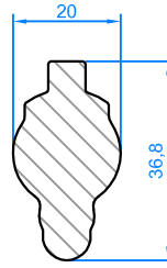
Pistol body Corps de pistolet
