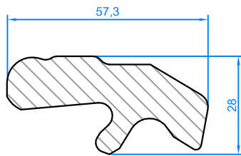
Profile for gun Profil pour fusil
