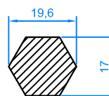
Doors torsion bar Leclerc tank Barre de torsion portes char Leclerc
