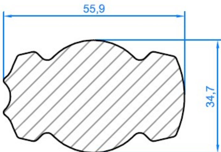
Profil pour transmission Profile for gear box Profil für Getriebe
