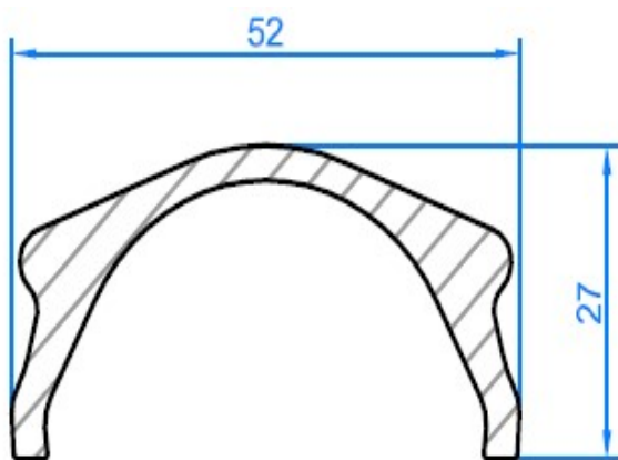
Colonne de direction, profil de guidage Slide way for steering column Gleitbahn für Lenksäule
