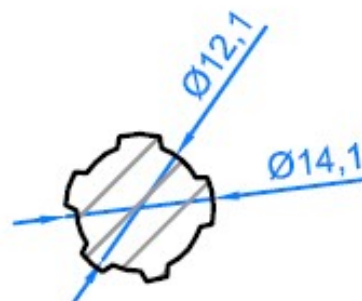
Ecrou antivol de roue Wheel lock nut Radsicherungsmutter
