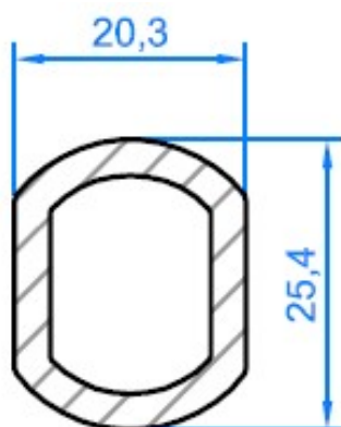
Colonne de direction « double D » Shaped form for steering column Lenksäule "Doppel-D"
