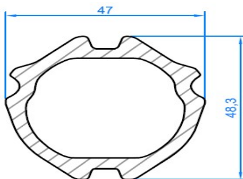
Colonne électrique, profil intérieur Electric column, interior profile Elektrische Säule, Innenprofil
