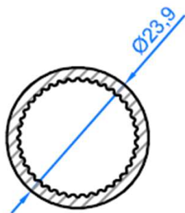
Tube cannelé de colonne de direction Splined shaft for steering column Keilwelle für Lenksäule
