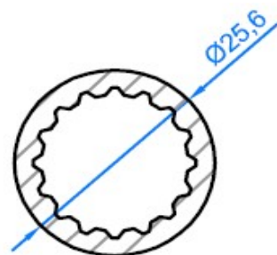
Tube cannelé de colonne de direction Splined shaft for steering column Keilwelle für Lenksäule
