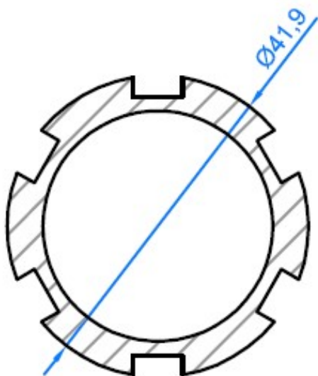
Colonne de direction, manchon antivol Anti-theft sleeve for steering column Anti-Diebstahl-Hülse für die Lenksäule
