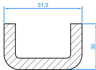
Rail for waste disposal vehicle Rail pour camion benne à ordures ménagères
