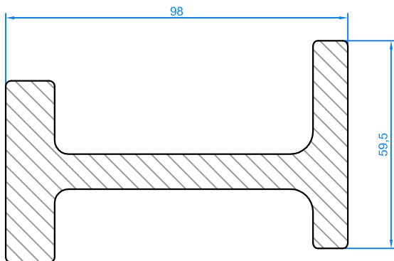
Fork lift section Profil pour chariot élévateur
