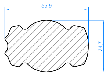
Profile for gear box Profil pour transmission
