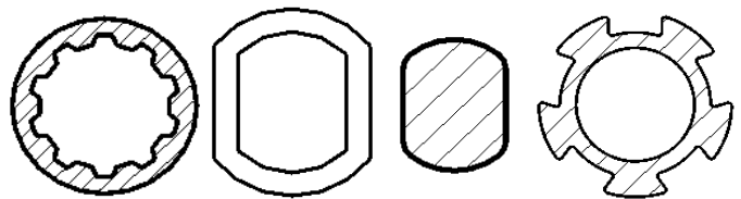
Tubes et profils pour colonnes de Direction Tubes and profiles for steering columns
